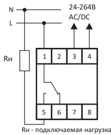
Схема подключения изделия и нагрузки, питающейся, от сети 230В.
